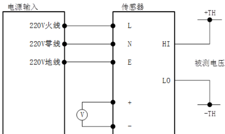
图 3 电气连接图
