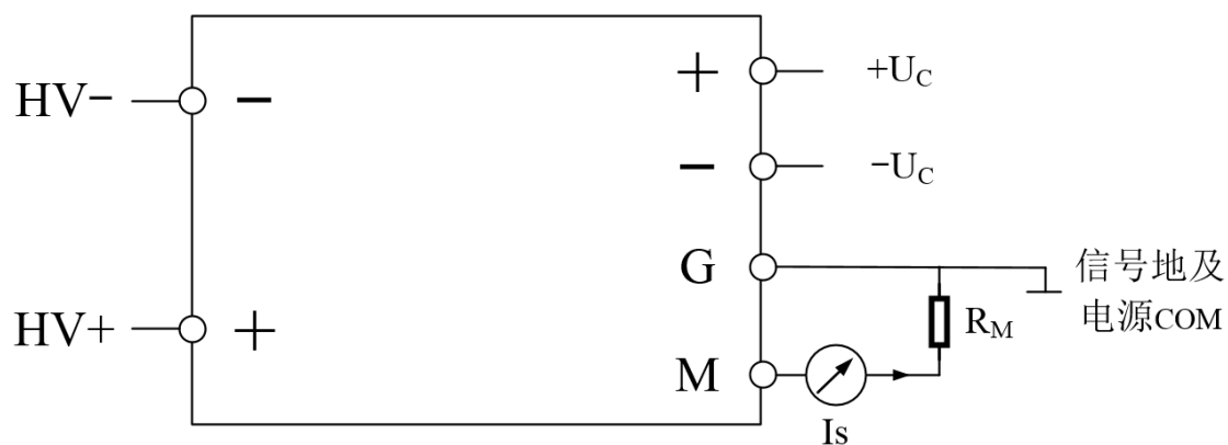
图 3 电气连接图
