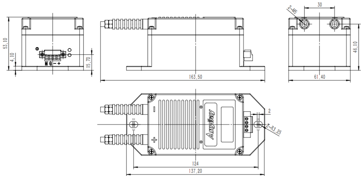
图 1 外形尺寸图
