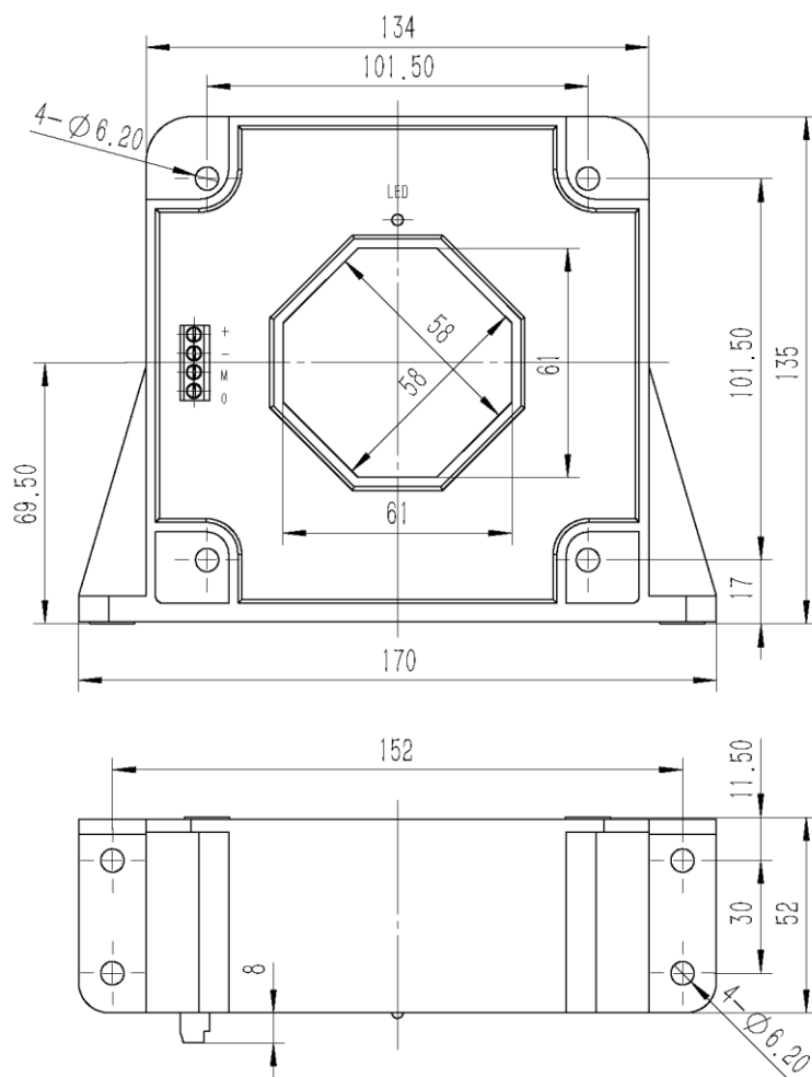
图 1 外形图
